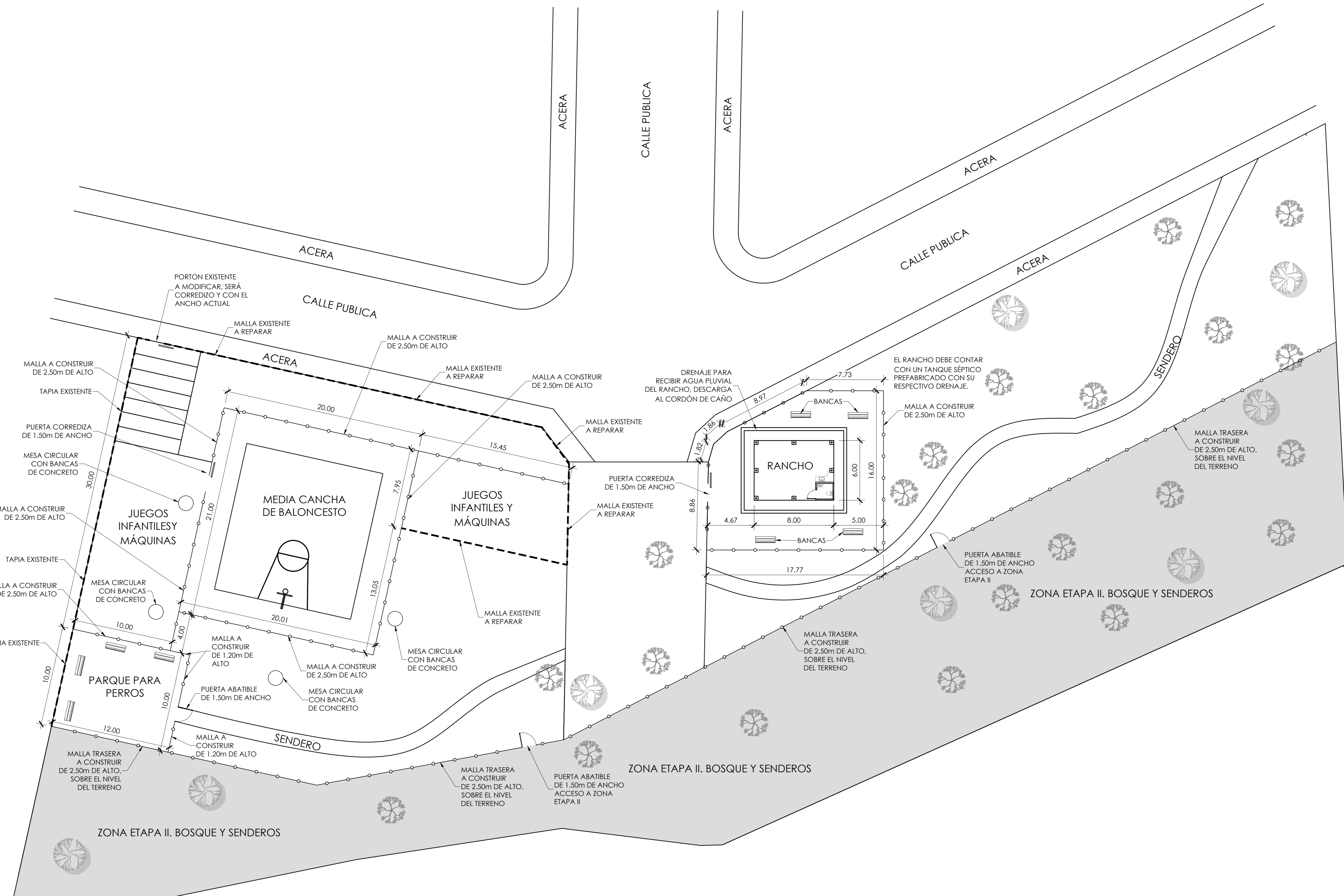
PLANTA DE CONJUNTO - PARQUE ECOLÓGICO VISTA REAL ESCALA 1:200
